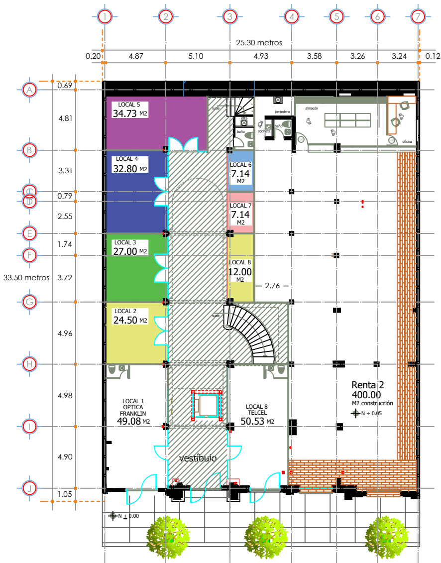
planta arquitectónica Planta Baja e s c a l a 1 : 1 0 0
